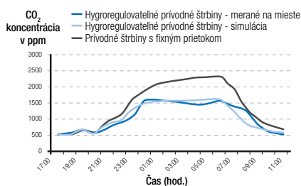
Obrázok 2: Zmeny CO 2 koncentrácií v spálni. Porovnanie hygro prívodných štrbín (merané a simulované) a štrbín s fixným prietokom (simulované).
